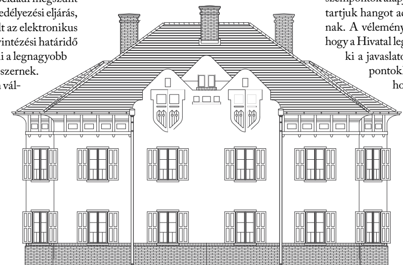
Az értékörzés alapja az eredeti kialakítás ismerete. Fleishl Róbert X. számú épülettípusának homlokzati rajza. Részlet a készülő Építészeti Kézikönyv II. kötetéből, rajz: Fazekas Csaba
