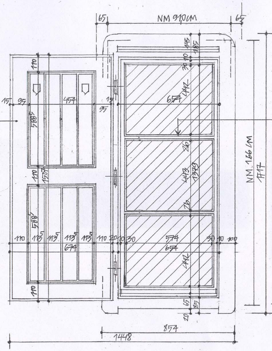
ABLAK HOMLOKZATI NÉZETE M=1:10
