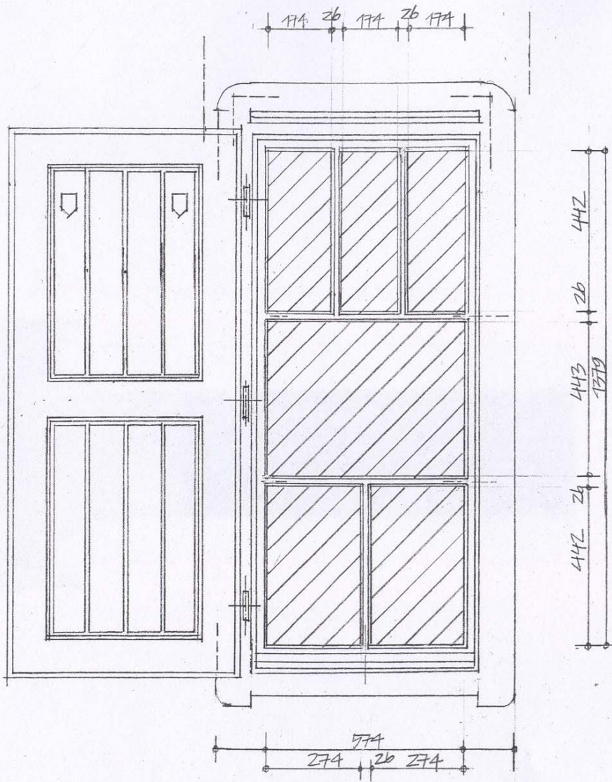
ABLAK HOMLOKZATI NÉZETE M=1:10 OSZTÓBORDA
