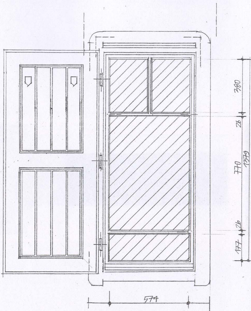
ABLAK HOMLOKZATI NÉZETE M=1:10 OSZTÓBORDA
