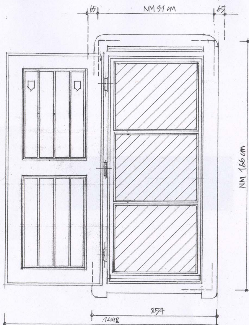
ABLAK HOMLOKZATI NÉZETE M=1:10
